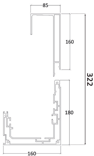
COURONNE SUR L'EXTENSION
