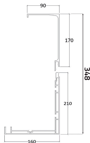
COURONNE SUR LA LARGEUR
