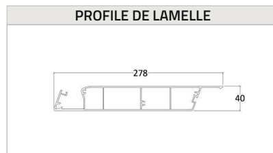
SEMI-OUVERT TOIT
